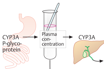
Ciclosporin
